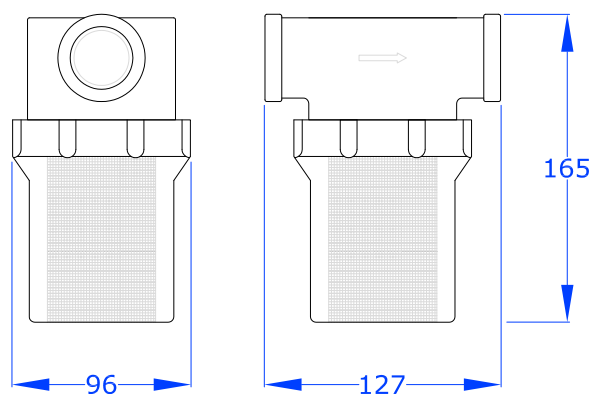
RV-ILS-1-T20E
