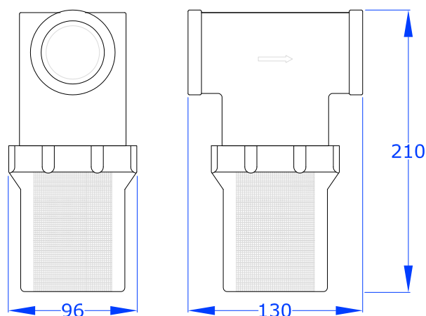
RV-ILS-1 1/2-T20E
