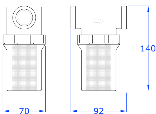
RV-ILS-3/4-T20E
