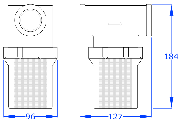
RV-ILS-1 1/4-T20E
