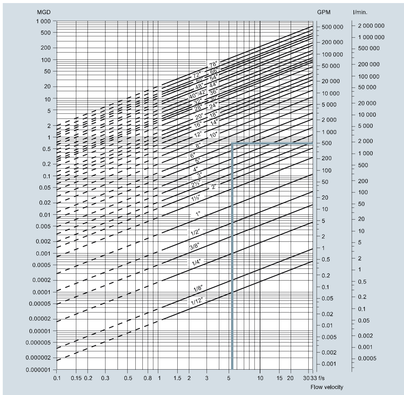
Sizing table ( 1/12'' ... 78'')
